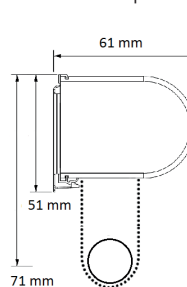
Malé nosiče pro 28 mm
